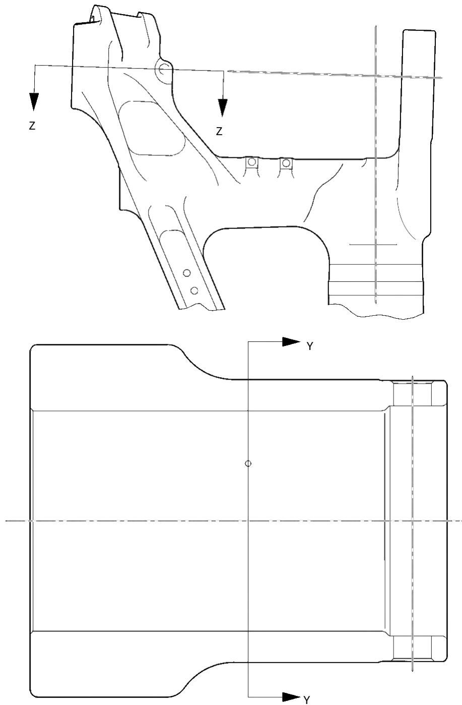
СЕЧЕНИЕ Z-Z
